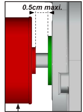
TOURILLON
